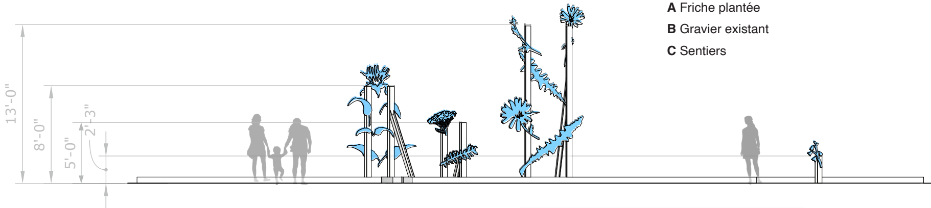
COUPE échelle 1/8" = 1' - 0" (1:96)
