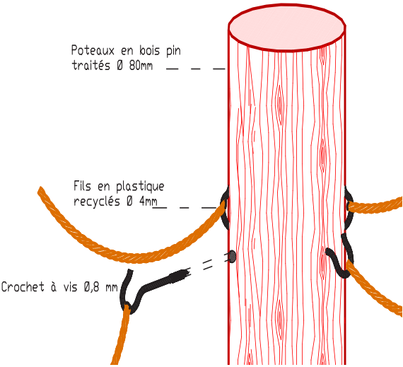
Détail schématique du poteau en bois
