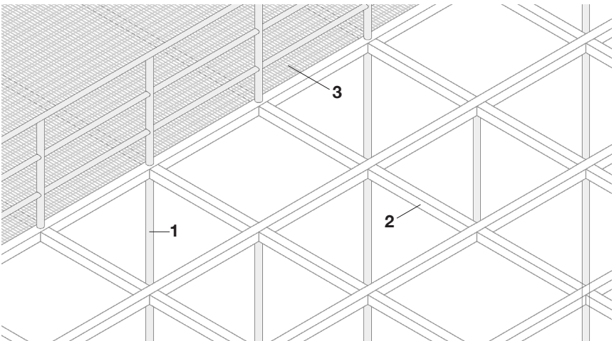
Assemblés comme des échafaudages à faible empreinte au sol, des tubes de métal chromé (1) soutiennent les quadrats en bois peint (2) et la passerelle en caillebotis (3).
