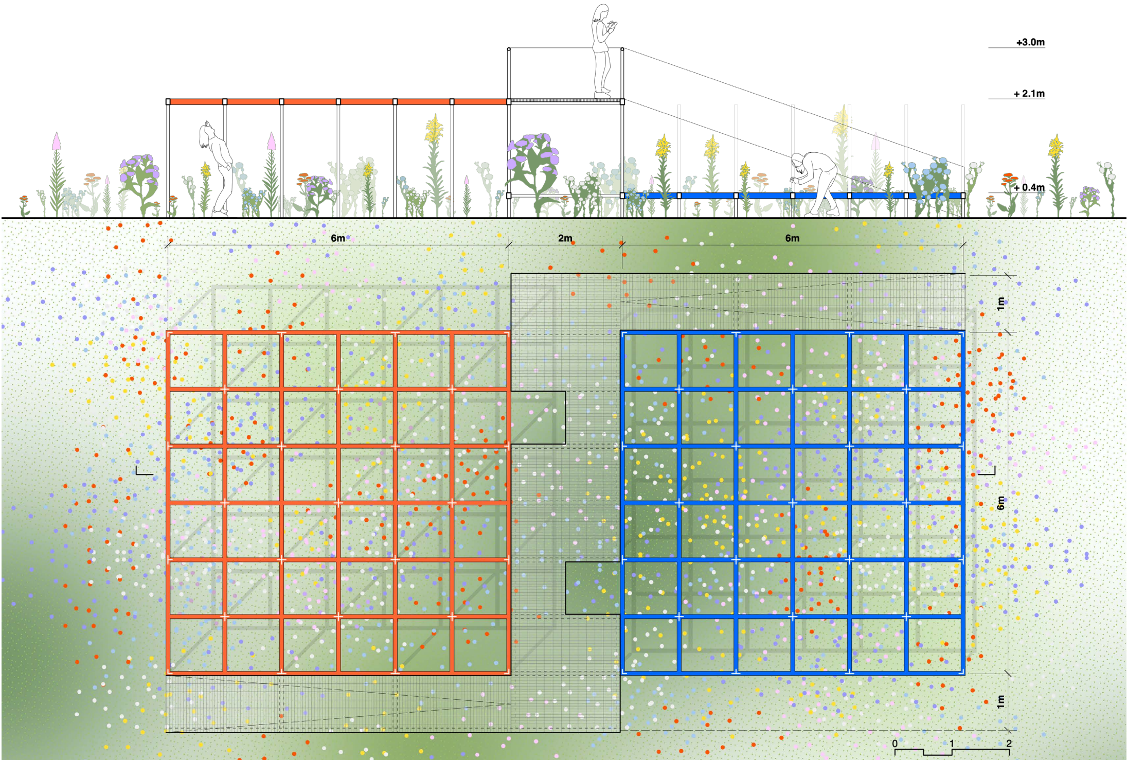
Plan et coupe
