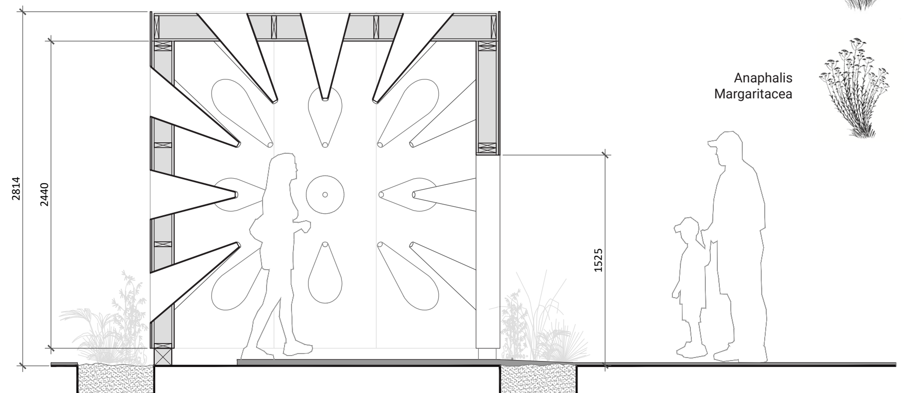
Coupe "A" du jardin - échelle 1 : 30
