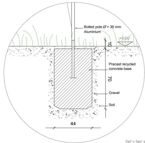
Det' c Sec' a'a
