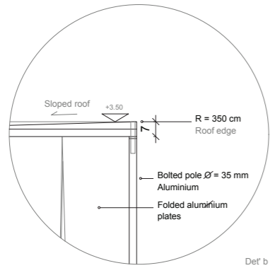
Det' b Sec' a'a
